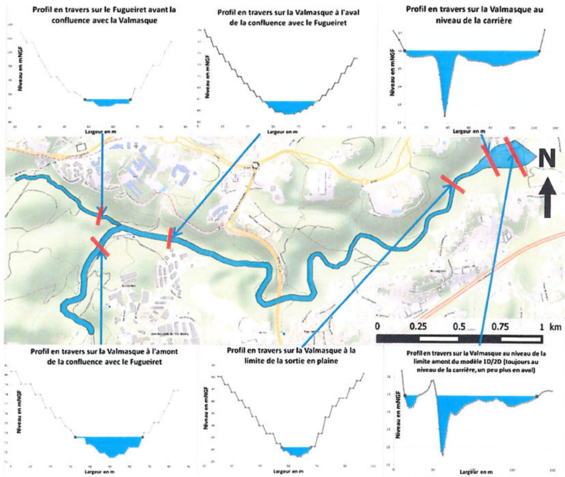
FIGURE 32 : EXEMPLE D'ANALYSE CAPACITAIRE SUR LA VALMASQUE AMONT
