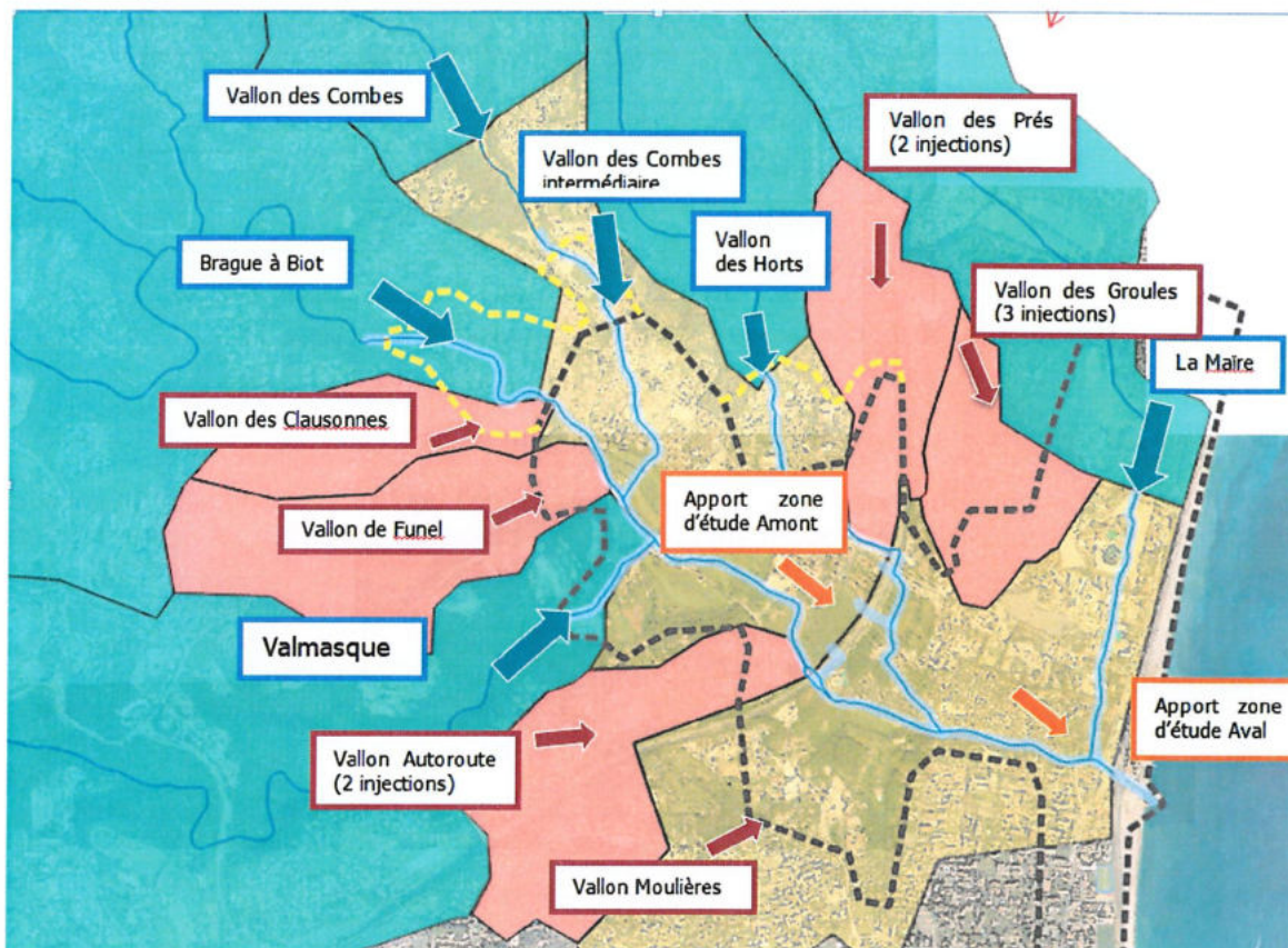
FIGURE 28 : INJECTION DES HYDROGRAMMES DANS LE MODÈLE 1D/2D
