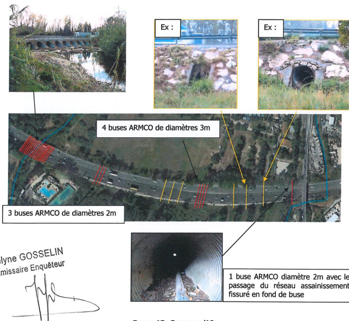
FIGURE 15 : BUSES DE L'A8
