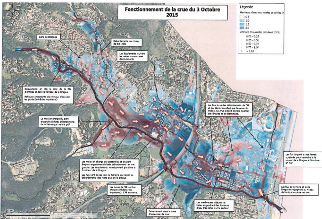
FIGURE 31 : FONCTIONNEMENT HYDRAULIQUE
