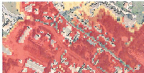
FIGURE 37 : RÉSULTATS DE SIMULATION SANS LES MURETS/HAIES DENSES - SECTEUR VAL DE PÔME
