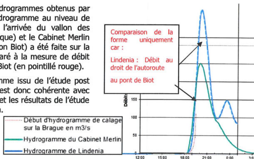
FIGURE 24 : COMPARAISON DES HYDROGRAMMES POUR LA CRUE DU 3 OCTOBRE 2015 SUR LA BRAGUE
