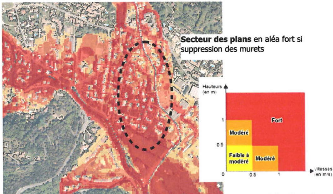
FIGURE 36 : RÉSULTATS DE SIMULATION SANS LES MURETS/HAIES DENSES - ALÉAS "BRUTS"
