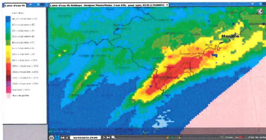
Cumul des précipitations en mm (lame d'eau Antilope), le 03/10 entre 20h et 23h. (La lame d'eau Antilope est une analyse combinée des données Radar et des pluviomètres)
